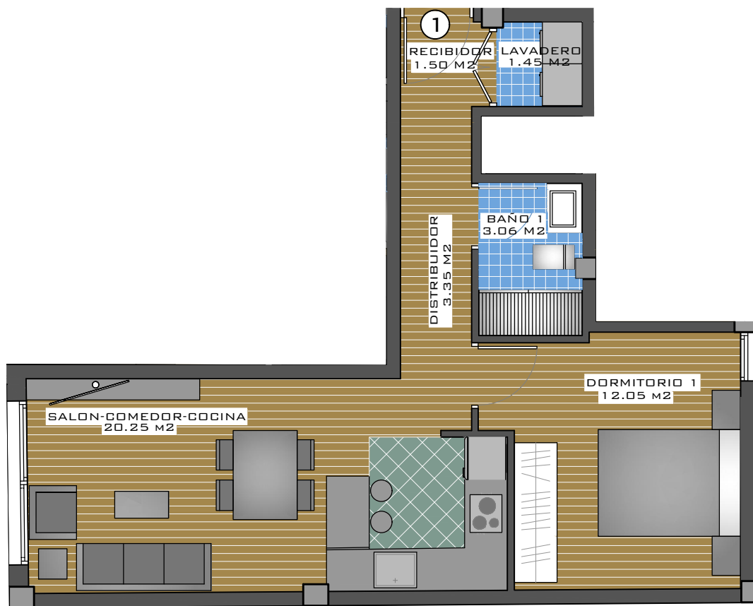
PLANTA TIPO
